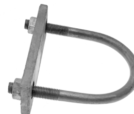
U-bult M16x112 mm Finns även i M12-76 mm och M12x112 mm
