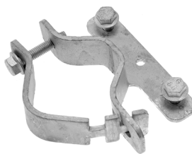
S-H klamma, enkel, galvad 48/60 mm Finns även i 76, 90, 108/114, 127/133, 152, 165, 180 mm
